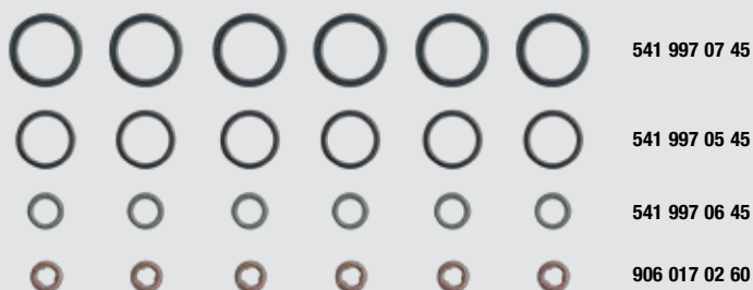
Illustration 2_OM 906 / OM 926, kit d'injecteurs 15-31357-03
